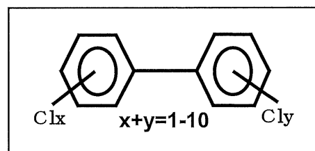
図1.1 PCBの構造
